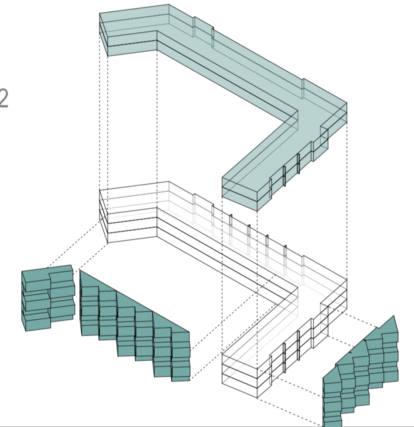
Ampliación de dos pisos, acoplamiento de cascaras que apuntan los departamentos al norte.
