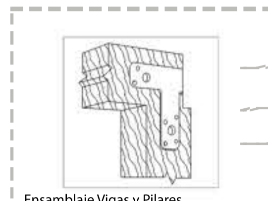
Ensamblaje Vigas y Pilares.
