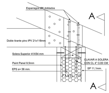
DETALLE APOYO TIPO ESCALA: 1/40
