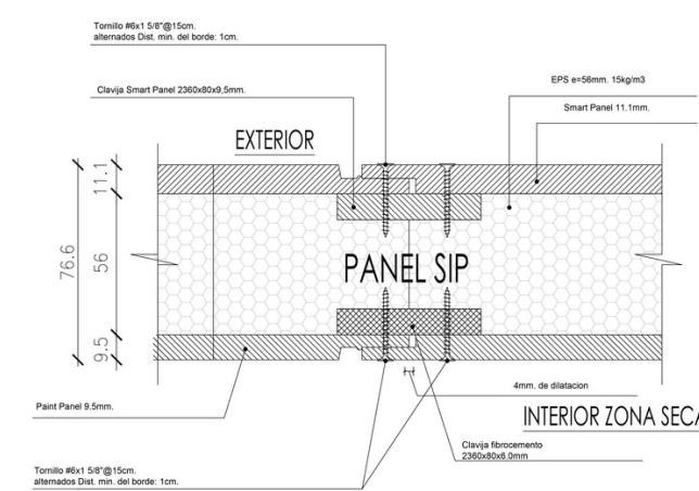
DETALLE DE UNION ESCALA: 1/40
