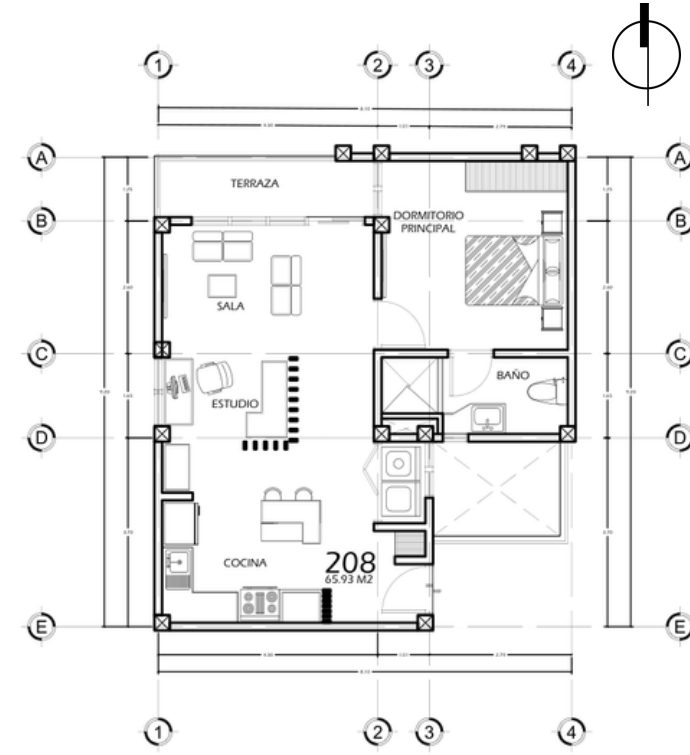
MÓDULO APARTAMENTO 1 - NIVEL 01 ESCALA: 1/100
