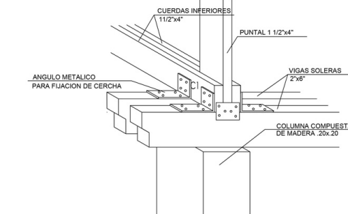
DETALLE DE UNION ESCALA: 1/40
