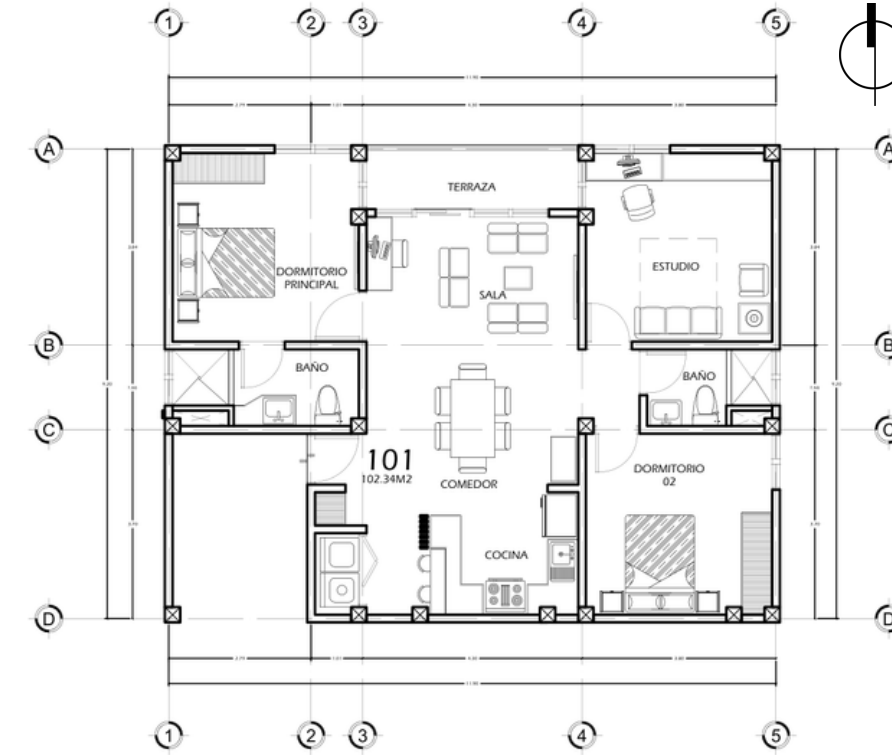
MÓDULO APARTAMENTO 2 - NIVEL 01 ESCALA: 1/100
