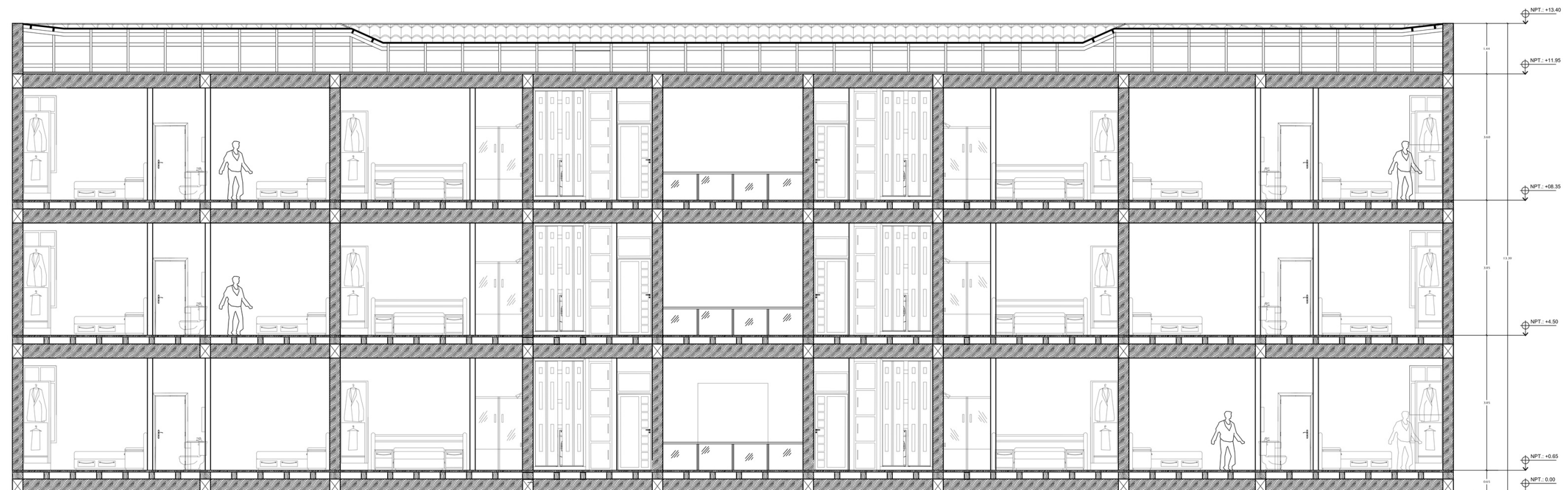
CORTE POR FACHADA ESCALA: 1/35
