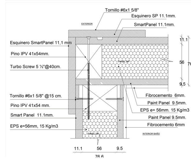
DETALLE DE UNION ESCALA: 1/40
