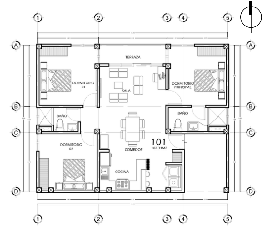
MÓDULO APARTAMENTO 3 - NIVEL 01 ESCALA: 1/100
