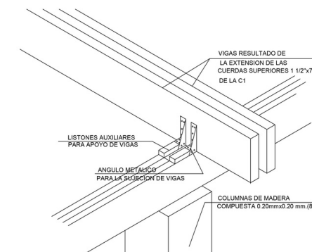
DETALLE DE UNION ESCALA: 1/40
