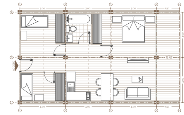
PLANTA SEGUNDO NIVEL | ESC 1:150
