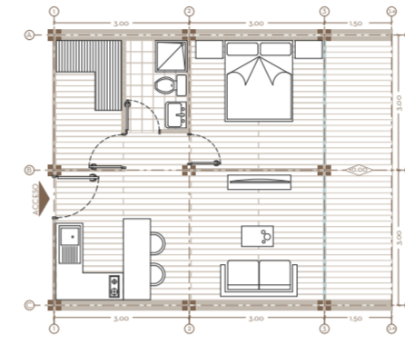
PLANTA PRIMER NIVEL HABITACIONAL | ESC 1:150
