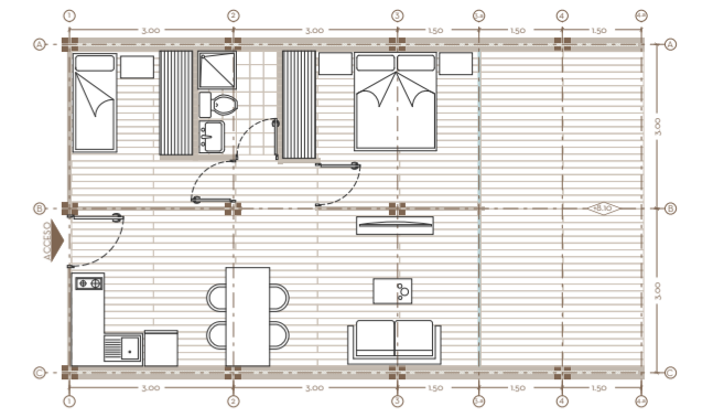
PLANTA CUARTO NIVEL | ESC 1:150
