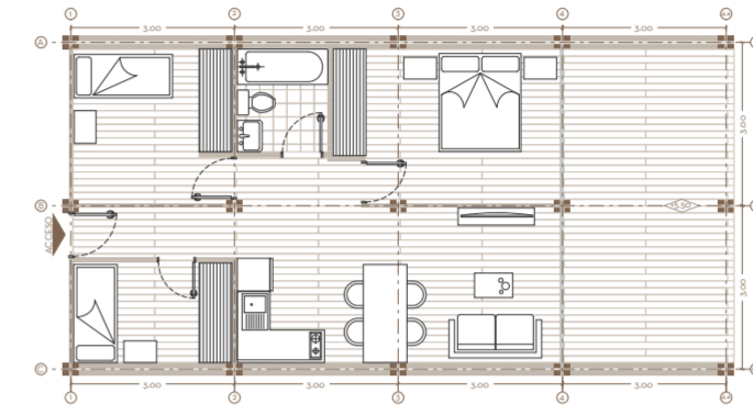
PLANTA TERCER NIVEL | ESC 1:150
