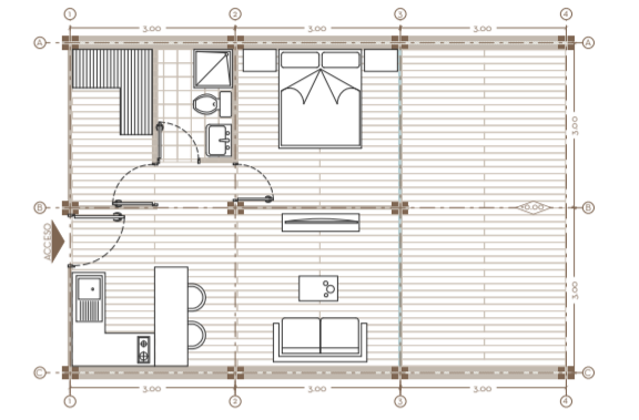
PLANTA QUINTO NIVEL | ESC 1:150
