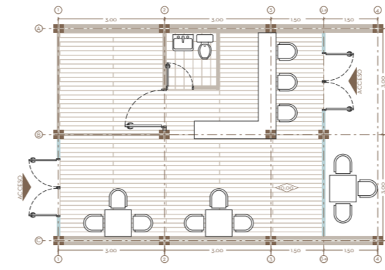
PLANTA PRIMER NIVEL COMERCIAL | ESC 1:150
