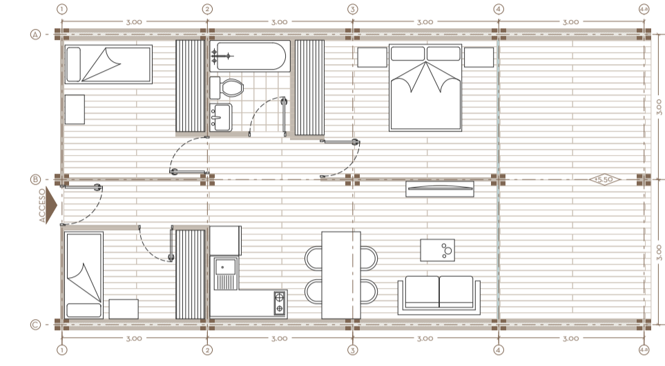
PLANTA TERCER NIVEL | ESC 1:100
