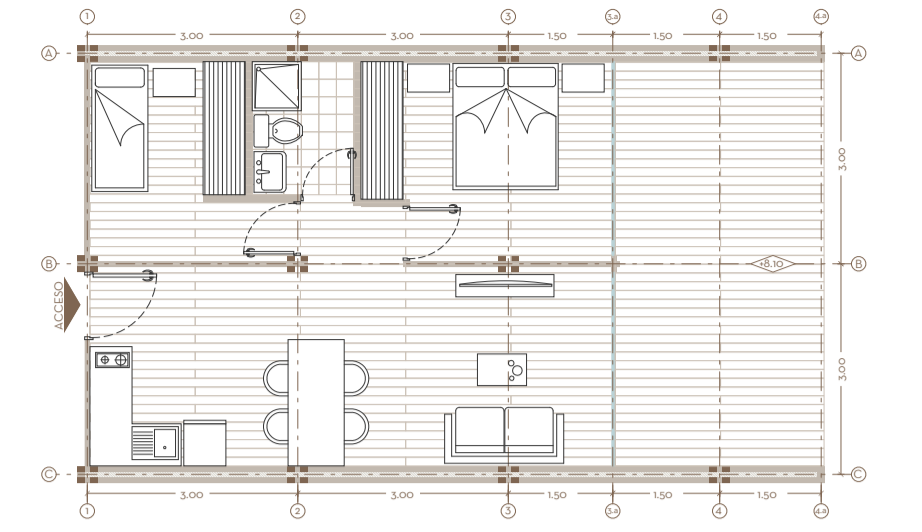
PLANTA CUARTO NIVEL | ESC 1:100
