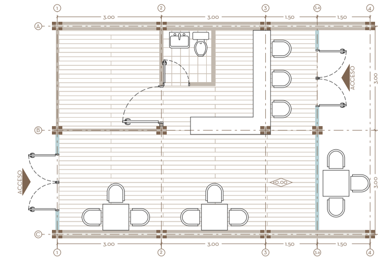
PLANTA PRIMER NIVEL COMERCIAL | ESC 1:100
