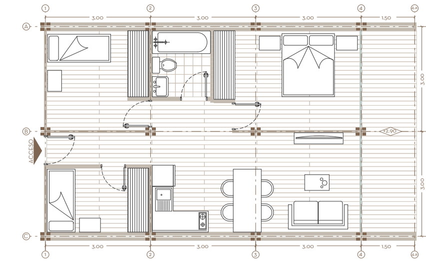
PLANTA SEGUNDO NIVEL | ESC 1:100
