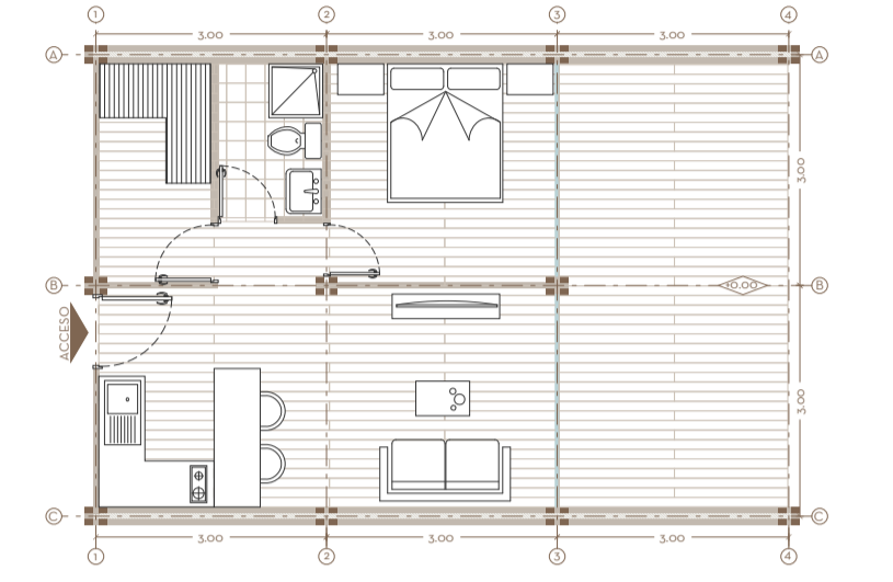
PLANTA QUINTO NIVEL | ESC 1:100
