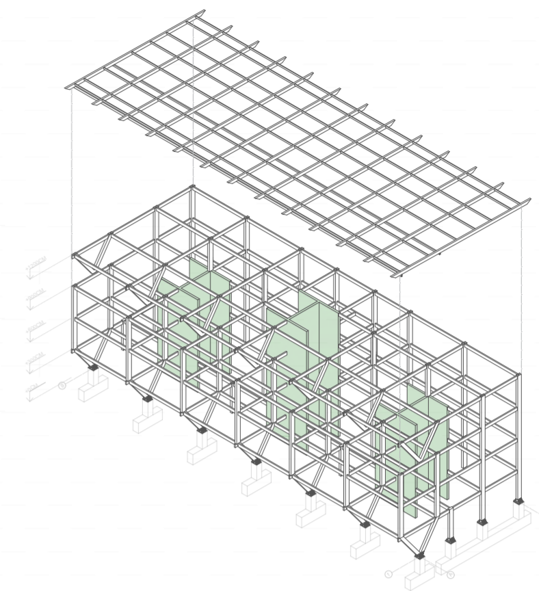
ESTRUCTURA PORTANTE / PILAR-MURO-VIGA
