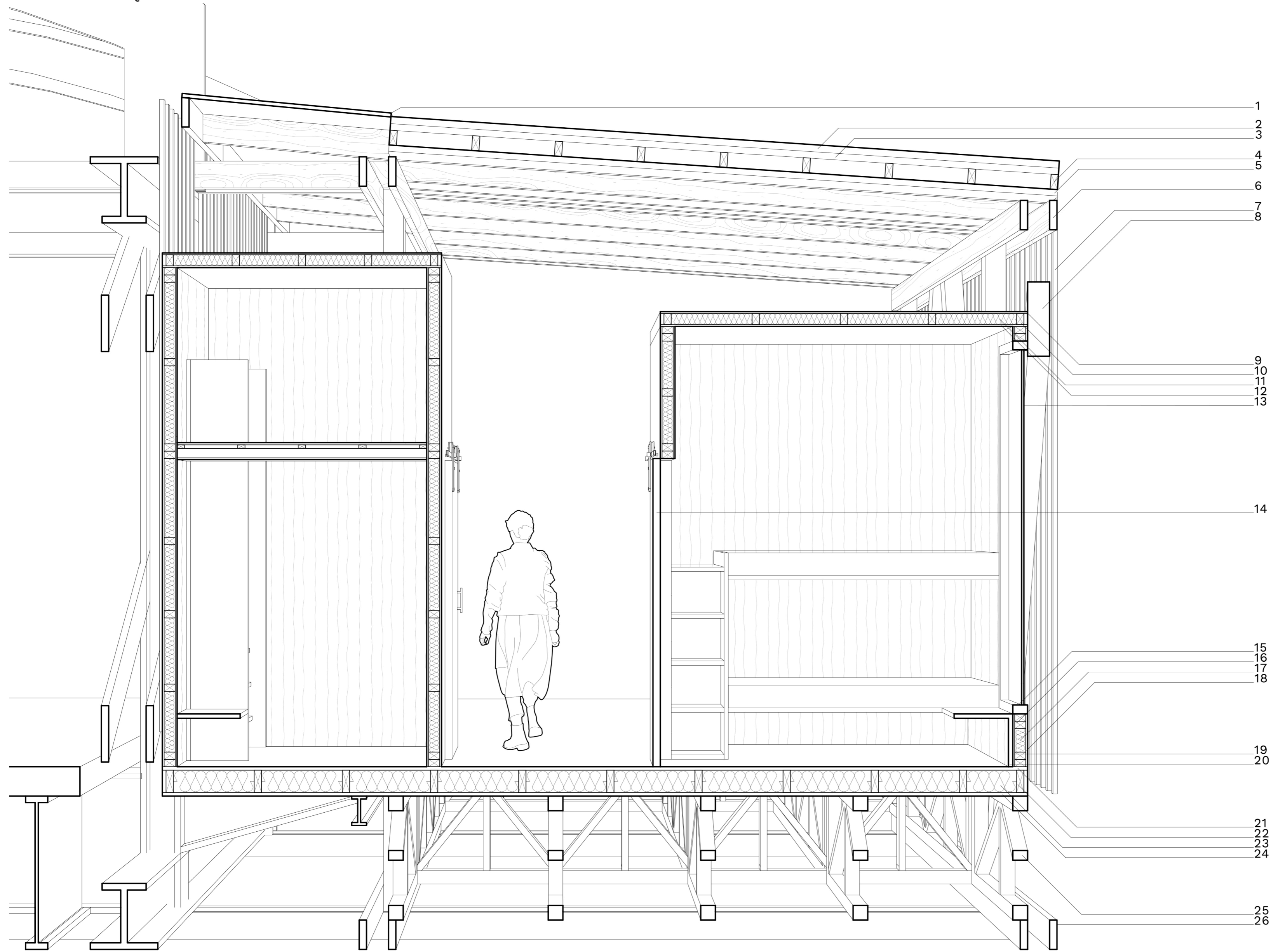
CORTE BB' CONSTRUCTIVO E. 1/20
