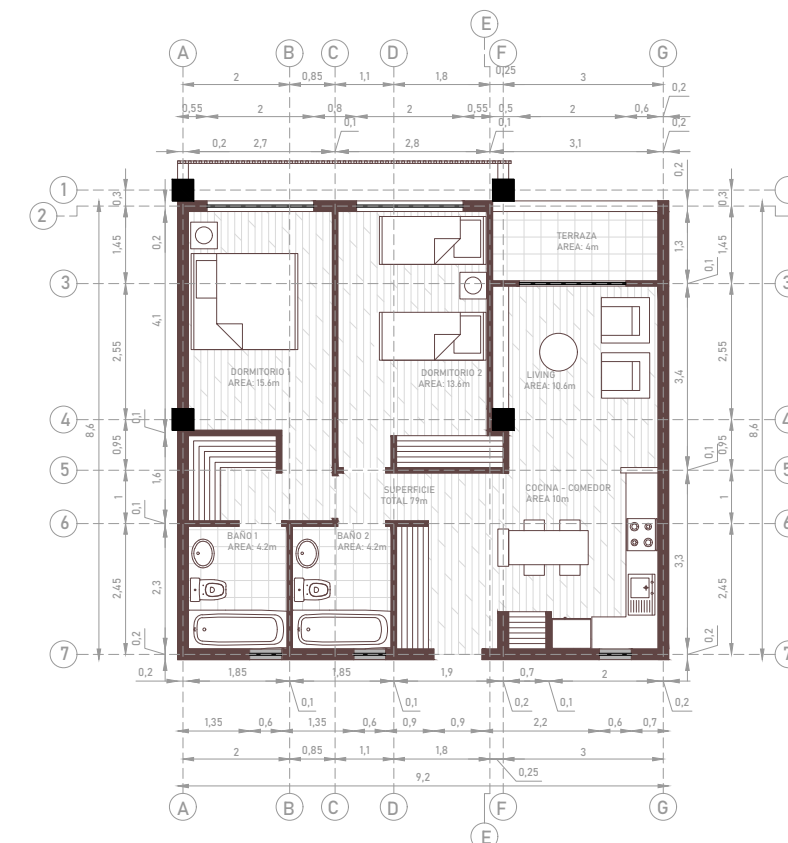
Planta TIPO A y B, 1:100
