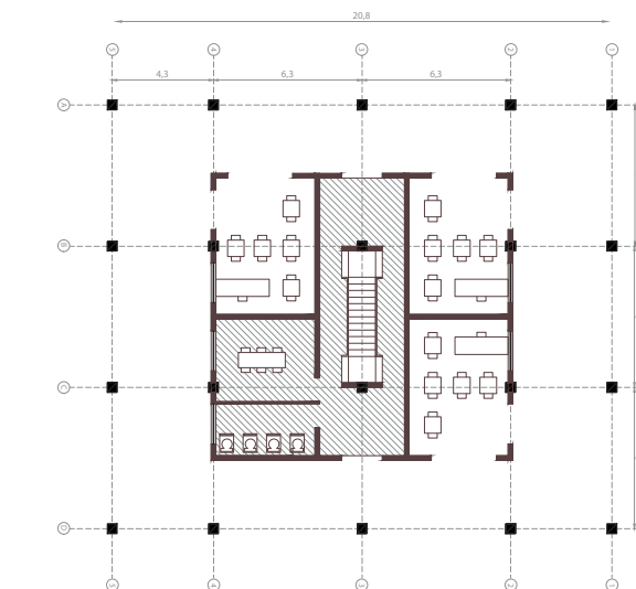
Planta nivel 1, 1:250
