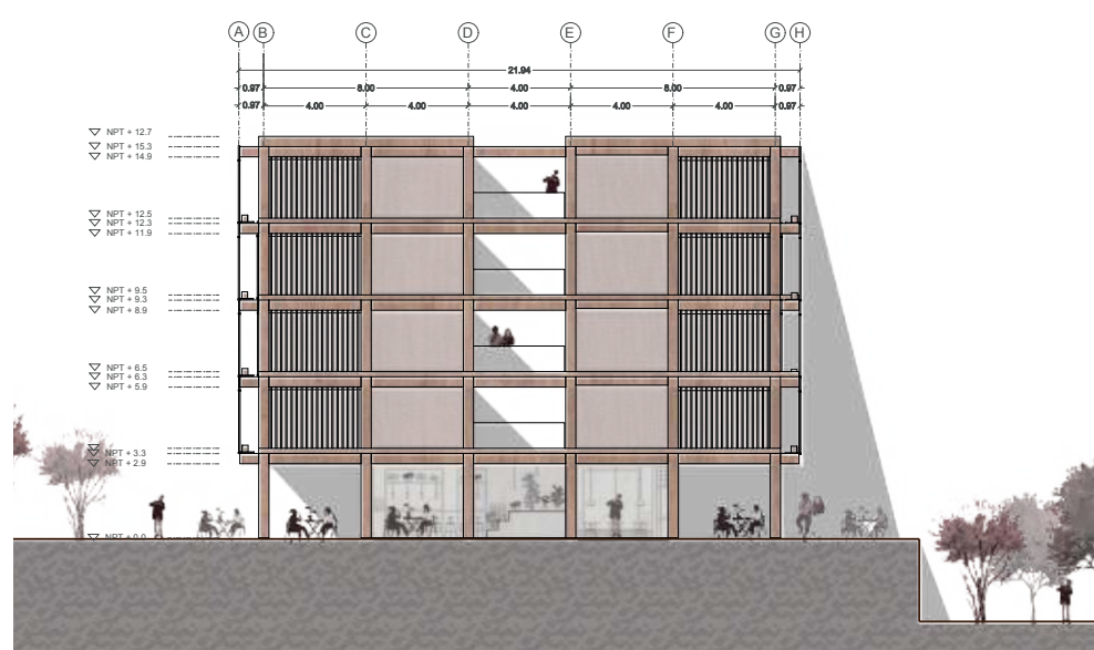
Elevacion fachada Oriente, 1:250
