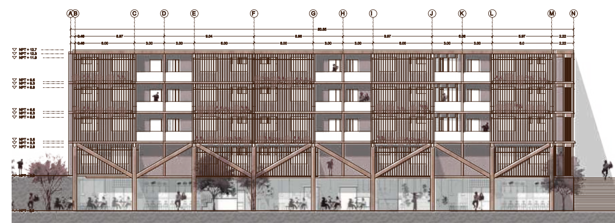
Elevacion fachada norte, 1:250
